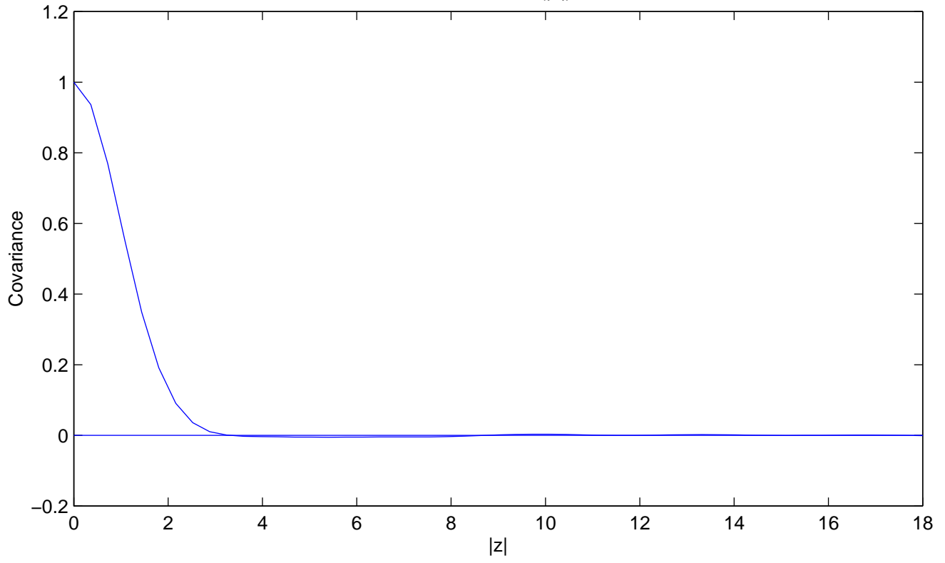
Covariance B(|z|)
